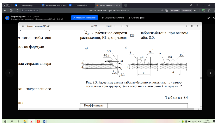
Рисунок 1.3 – Расчетные схемы набрызг-бетонного покрытия: а — самостоятельная конструкция; б — в сочетании с анкерами 1 и арками 2
