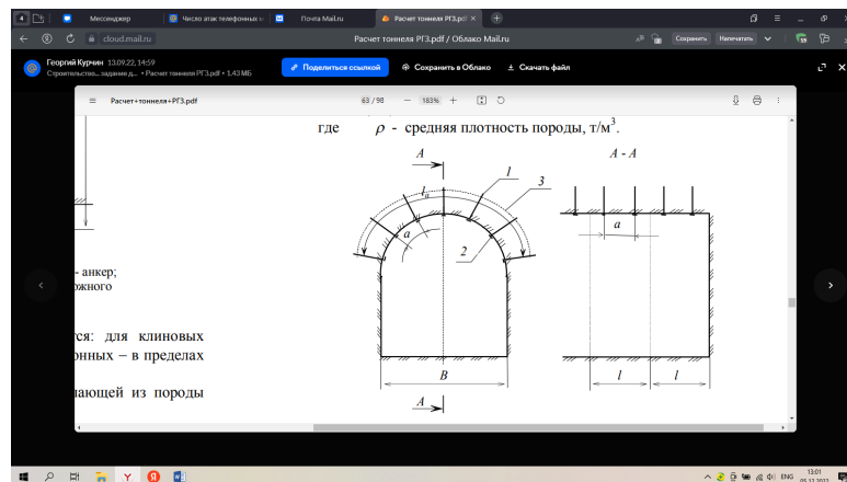
Рисунок 1.2 – Схема к расчету анкеров на заходку
