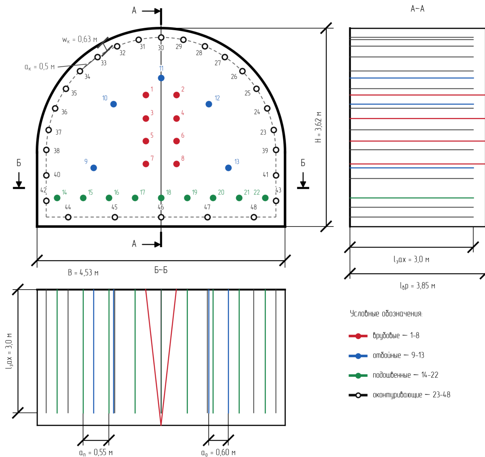
Рисунок 2.1 – Схема расположения шпуров
