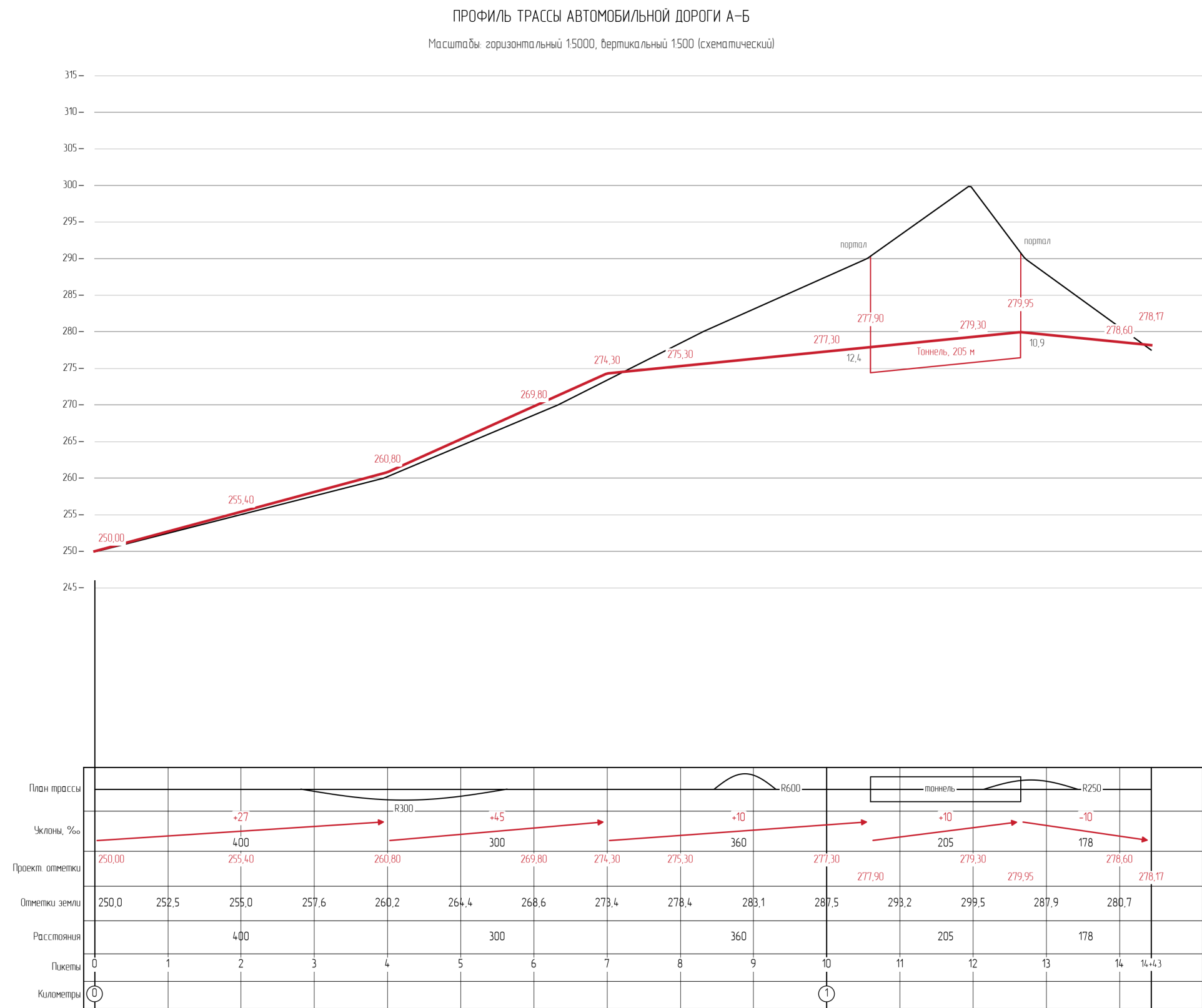
Рисунок 2.3 – Профиль трассы (масштабы: горизонтальный 1:5000, вертикальный 1:500)
