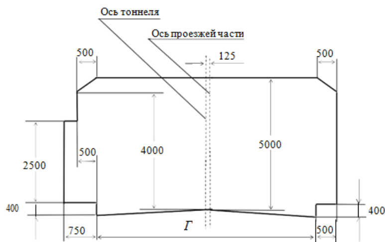
Рисунок 1.2 – Габарит приближения строений и оборудования для дорог III и IV категорий Ширина проезжей части \Gamma приведена в Таблице 1.1.
