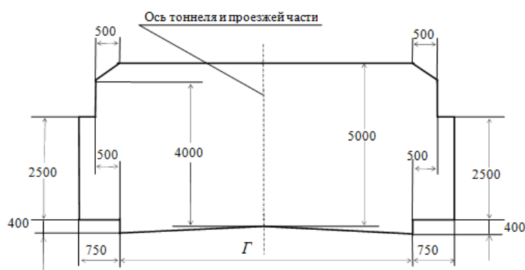
Рисунок 1.1 – Габарит приближения строений и оборудования для дорог I и II категорий
