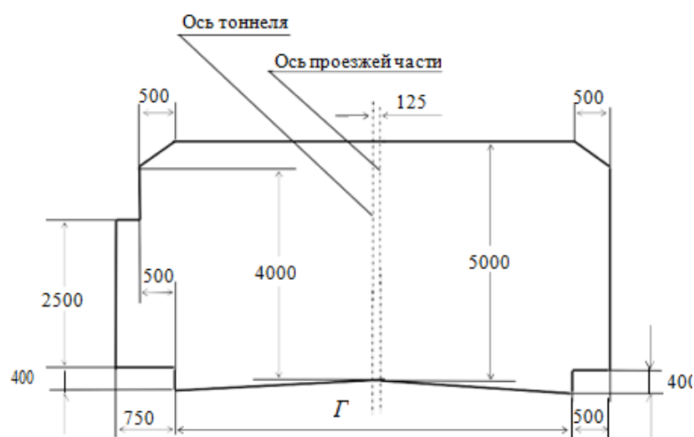
Рисунок 2 — Габарит приближения строений и оборудования для дорог III и IV категорий
