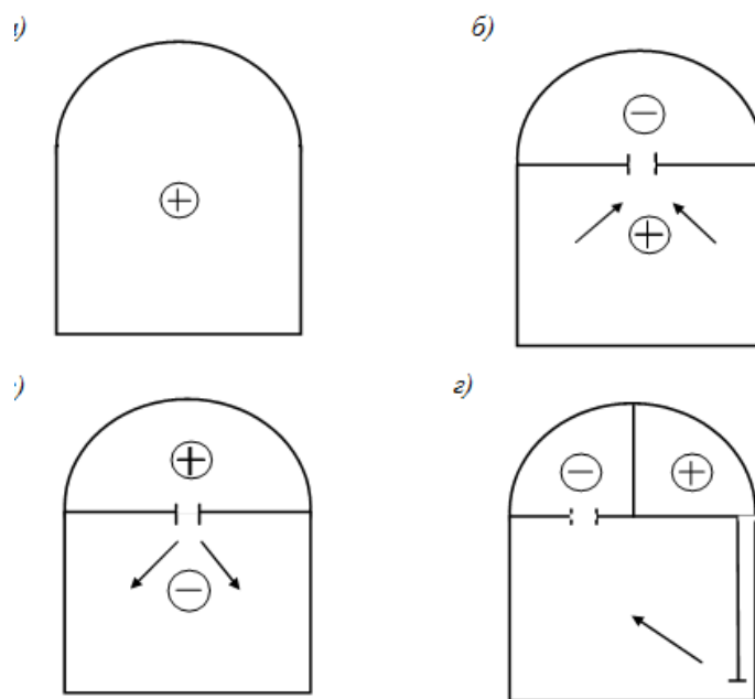
Рисунок 3 — Системы искусственной вентиляции в тоннелях: а — продольная; б — полупродольная; в — полупоперечная; г — поперечная; + — движение свежего воздуха; — — движение отработанного воздуха
