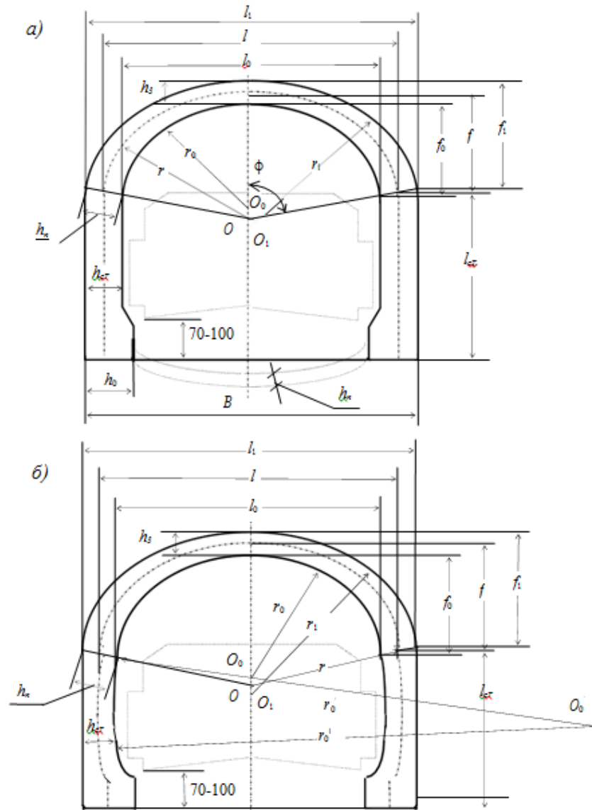
Рисунок 4 — Конструирование свода обделки: а — пологого свода; б — подъемистого свода
