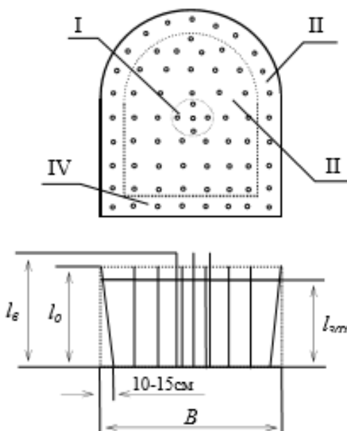
Рисунок 1.1 – Группы шпуров в забое: I — врубовые; II — отбойные; III — контурные; IV — подошвенные; B — ширина выработки; l_{\text{в}} — глубина врубовых шпуров; l_{\text{от}} — глубина отбойных шпуров; l_{\text{зах}} — величина заходки
