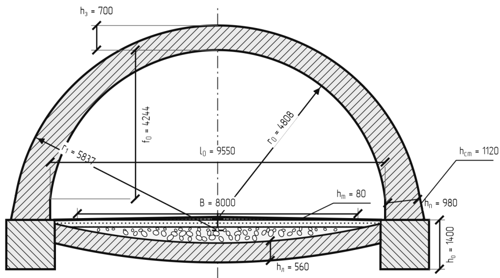
Рисунок 2.1 – Поперечное сечение обделки
