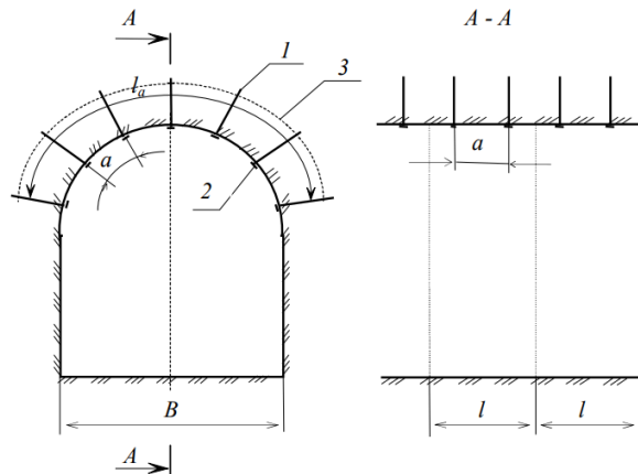
Рисунок 1.2 – Схема к расчету анкеров на заходку
