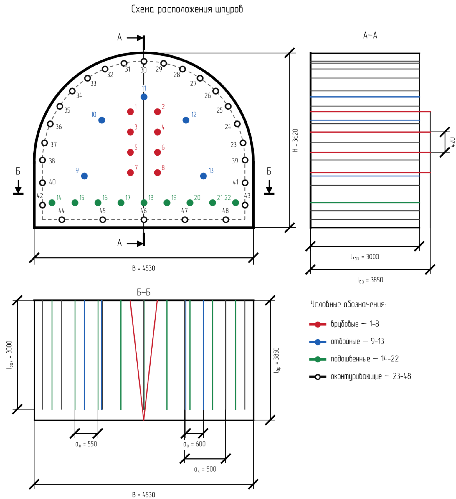
Рисунок 2.1 – Схема расположения шпуров
