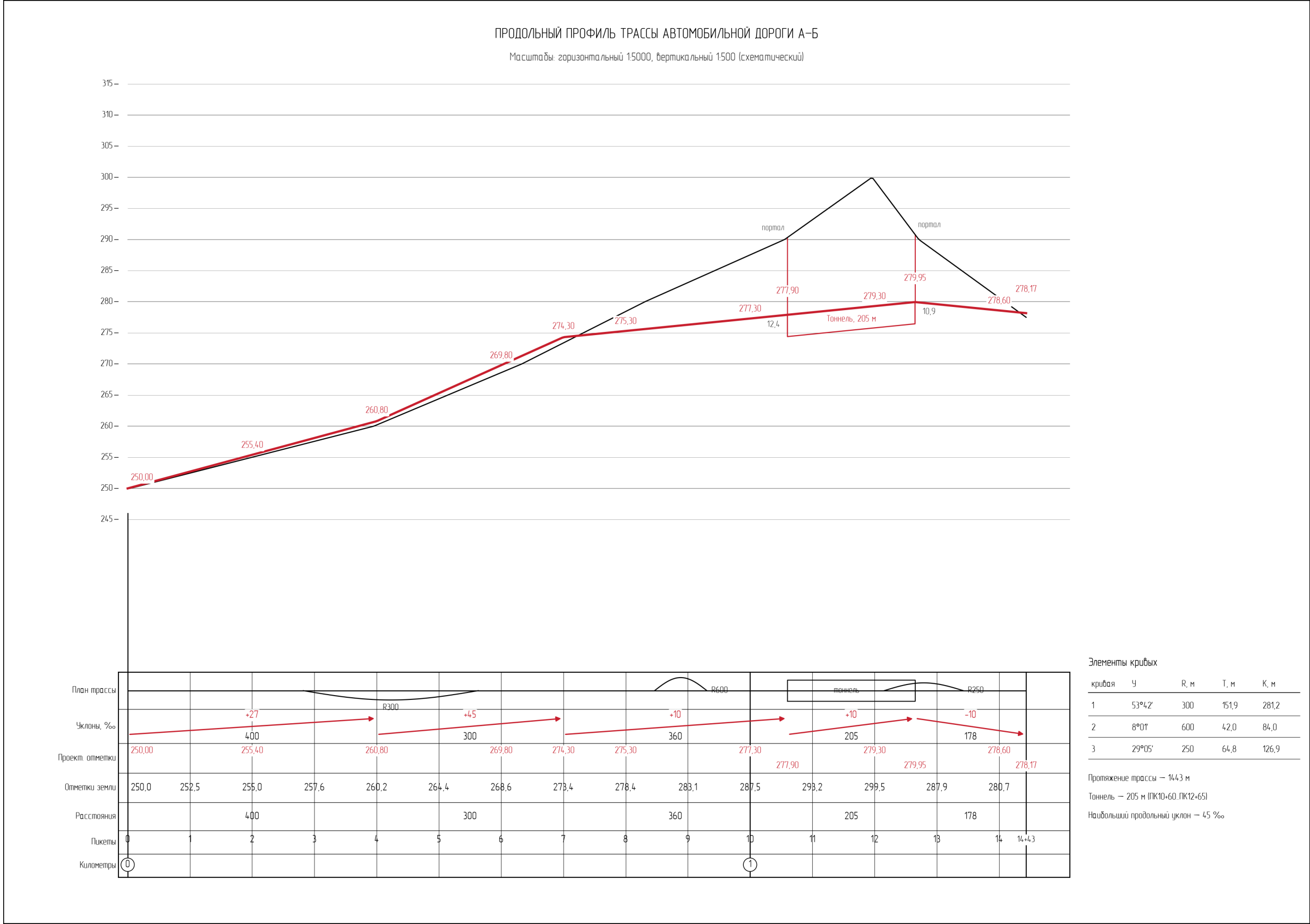
Рисунок 2.3 – Продольный профиль трассы (масштабы: горизонтальный 1:5000, вертикальный 1:500)
