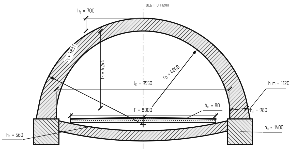
Рисунок 2.1 – Поперечное сечение обделки подъемистого очертания с обратным сводом
