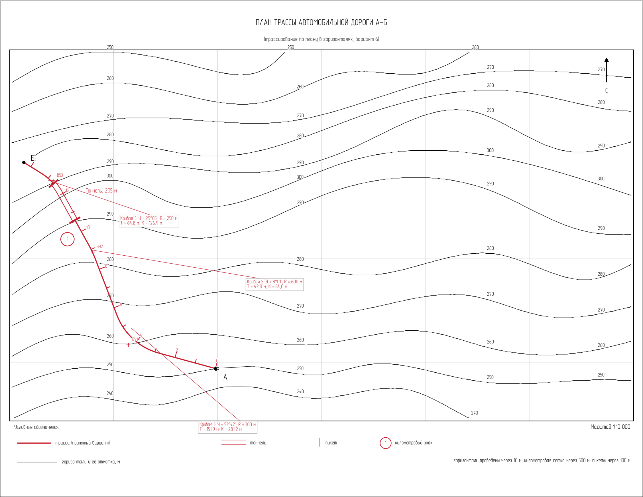
Рисунок 2.2 – План трассы автомобильной дороги от пункта А до пункта Б: циркульный ход с шагом 1,11 см, кривые радиусами 250...600 м, тоннель длиной 205 м у водораздела
