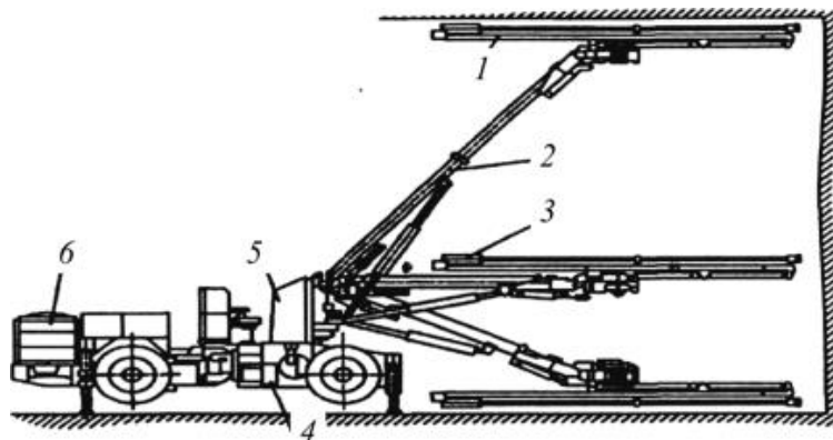
Рисунок 1.1 – Шахтная бурильная установка: 1 — податчик; 2 — манипулятор; 3 — бурильная головка; 4 — рама с ходовой частью; 5 — пульт и система управления; 6 — привод
