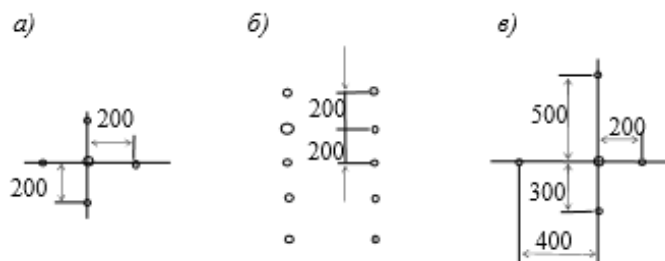
Рисунок 1.3 – Дробящие (прямые) врубы: а — призматический; б — щелевой; в — спиральный
