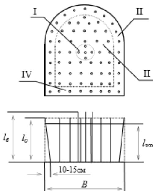
Рисунок 1.1 – Группы шпуров в забое: I — врубовые; II — отбойные; III — контурные; IV — подошвенные; B — ширина выработки; l_{\text{в}} — глубина врубовых шпуров; l_{\text{o}} — глубина отбойных шпуров; l_{\text{зах}} — величина заходки
