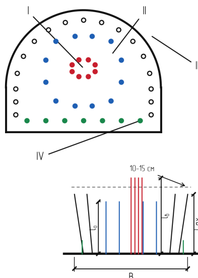
Рисунок 1.1 – Группы шпуров в забое: I — врубовые; II — отбойные; III — контурные; IV — подошвенные; B — ширина выработки; l_v — глубина врубовых шпуров; l_o — глубина отбойных шпуров; l_{зax} — величина заходки
