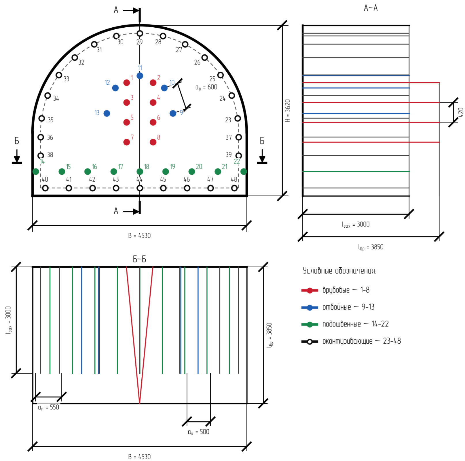
Рисунок 2.1 – Схема расположения шпуров
