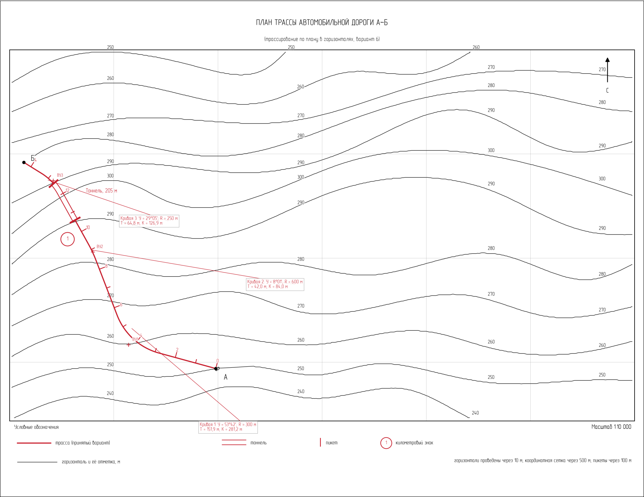
Рисунок 2.2 – План трассы автомобильной дороги
