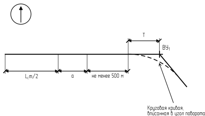
Рисунок 1.1 – Начало трассирования
